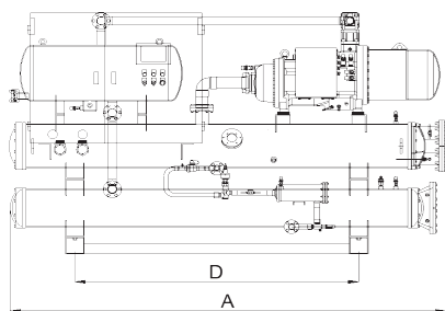
PQDF-K140/PQDF-K175/PQDF-K210
