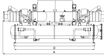
PQDF-K1260/PQDF-K1400
