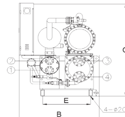
PQDF-K280/PQDF-K350/PQDF-K420
