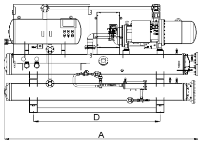
PQDF-K140/PQDF-K175/PQDF-K210
