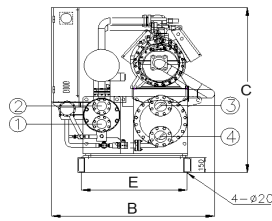
PQDF-K840/PQDF-K1050/PQDF-K1750/PQDF-K2100
