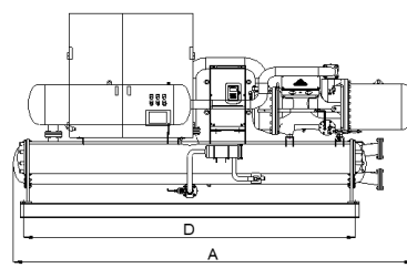
PQDF-K280/PQDF-K350/PQDF-K420
