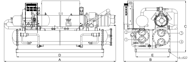
PQDF-K1260/PQDF-K1400/PQDF-K1750
