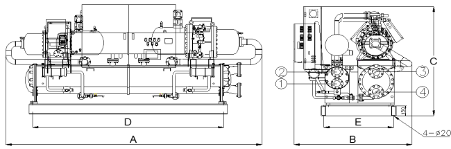
PQDF-K840/PQDF-K1050/PQDF-K2100
