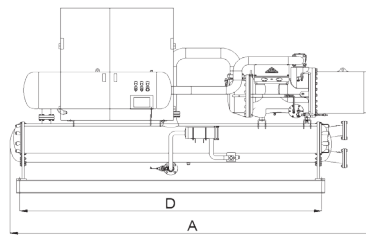
PQDF-K280/PQDF-K350/PQDF-K420
